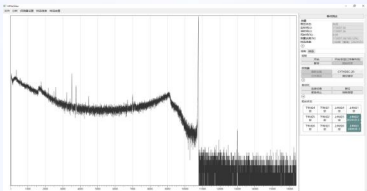
(软件主界面)
