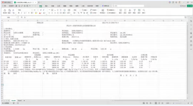
(导出报告)
